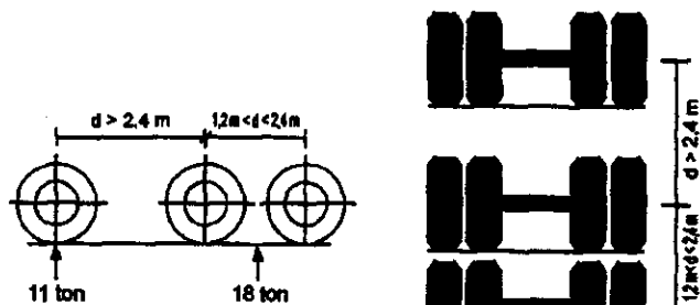
TRES EJES SIMPLES DISTANCIADOS 2 rodado doble, mas 1 rodado doble distanziado a mas de 2,4 m (2RD + 1RD)
