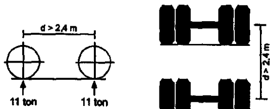
DOS EJES SIMPLES DISTANCIADOS Rodado doble, más rodado doble distanziado a más de 2,4 m. c/u (1RD + 1RD)
