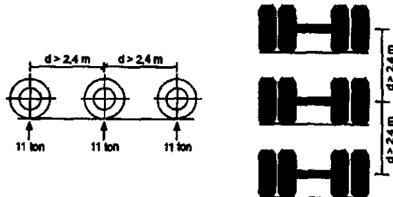
TRES EJES SIMPLES DISTANCIADOS Rodado doble, más rodado doble, más rodado doble, distanziado a mas de 2,4 m c/u (1RD + 1RD + 1RD)
